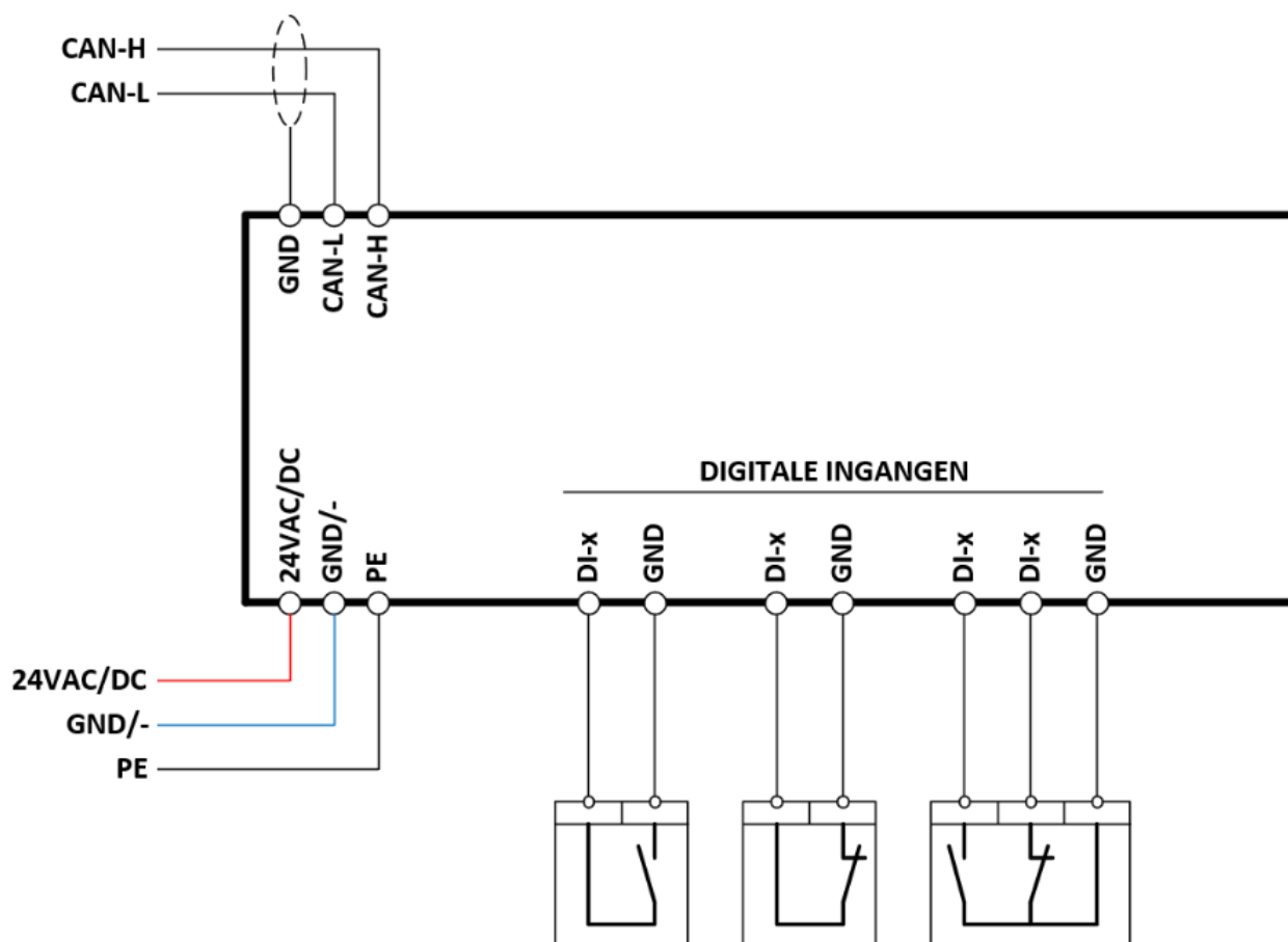
Figuur 2: Aansluitingen
