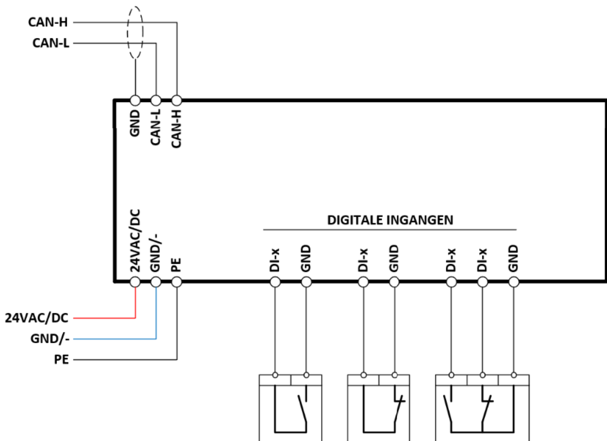
Figuur 2: Aansluitingen
