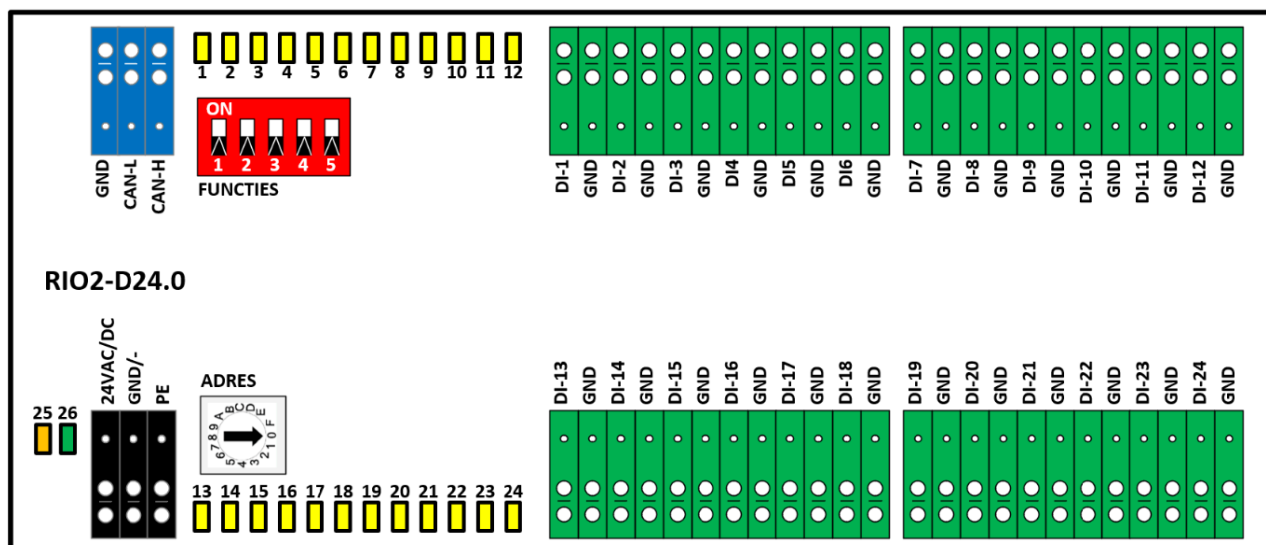
Figuur 1: Overzicht
