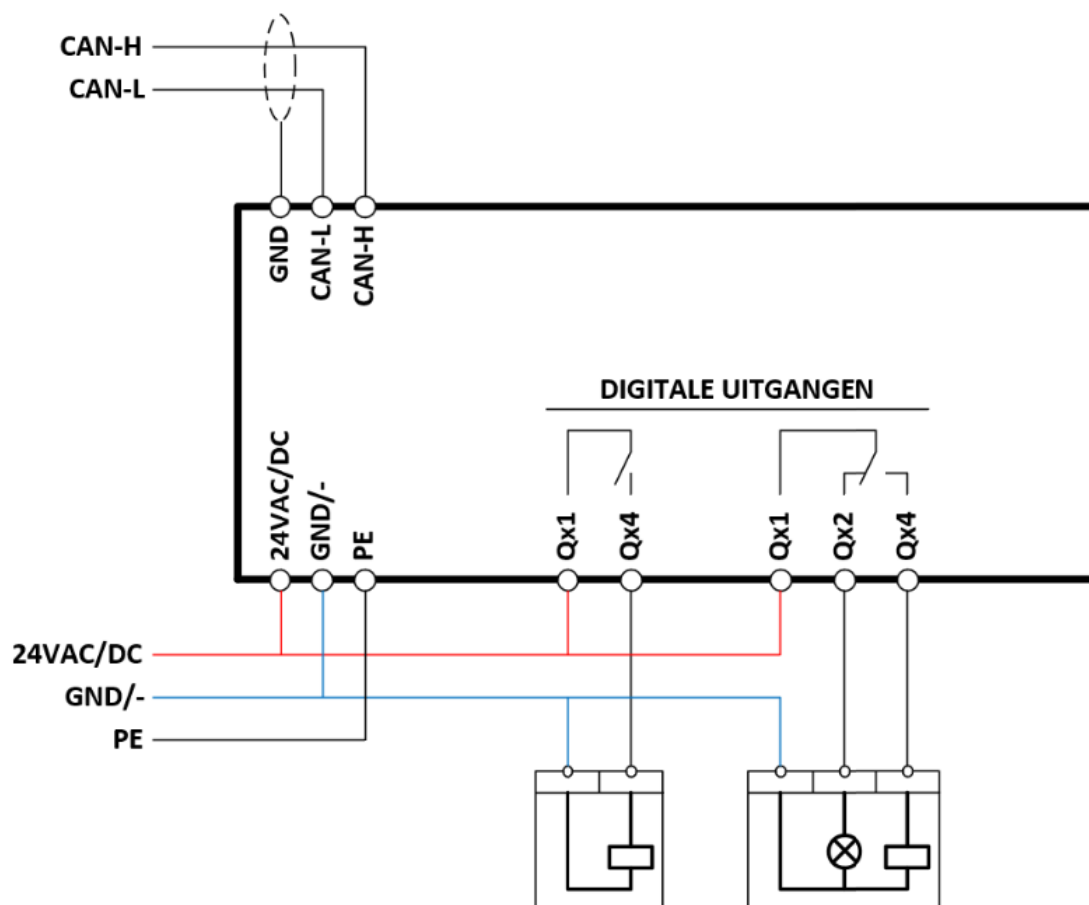
Figuur 2: Aansluitingen
