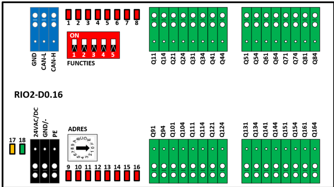
Figuur 1: Overzicht
