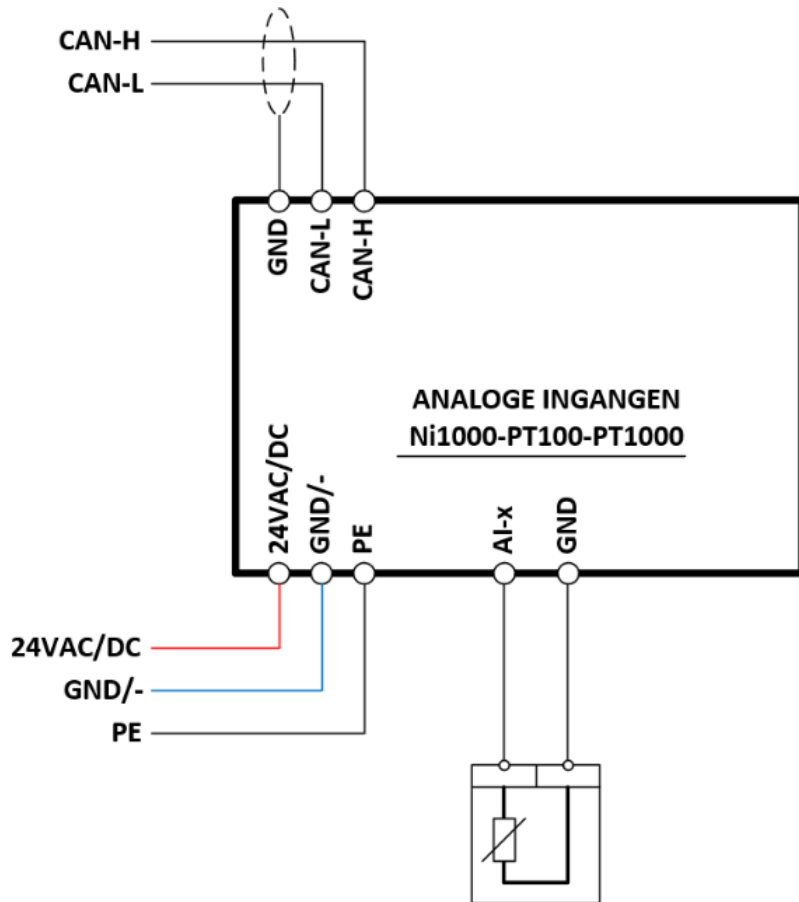
Figuur 2: Aansluitingen
