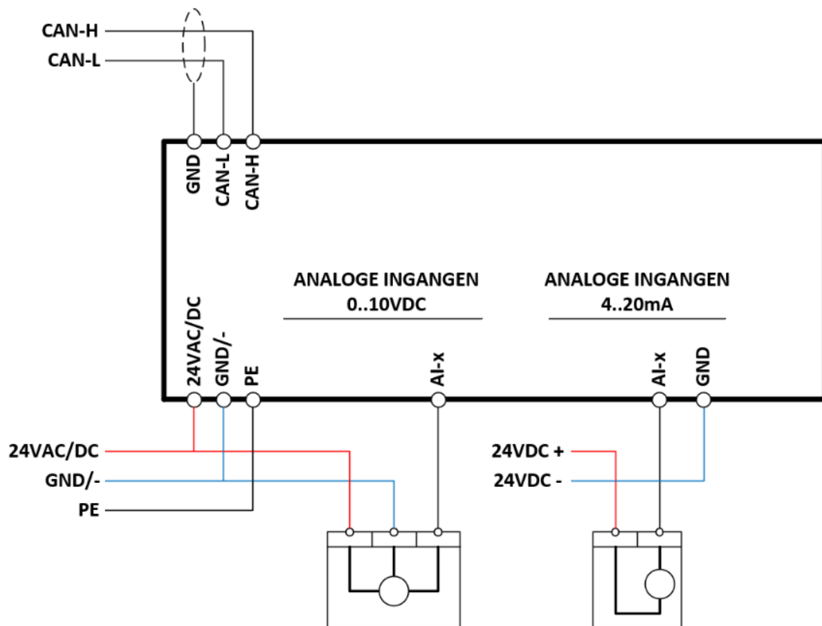
Figuur 3: Aansluitingen Analoge Ingangen
