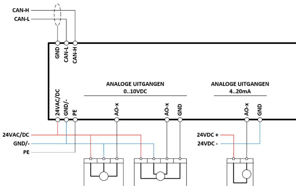
Figuur 3: Aansluitingen Analoge Uitgangen
