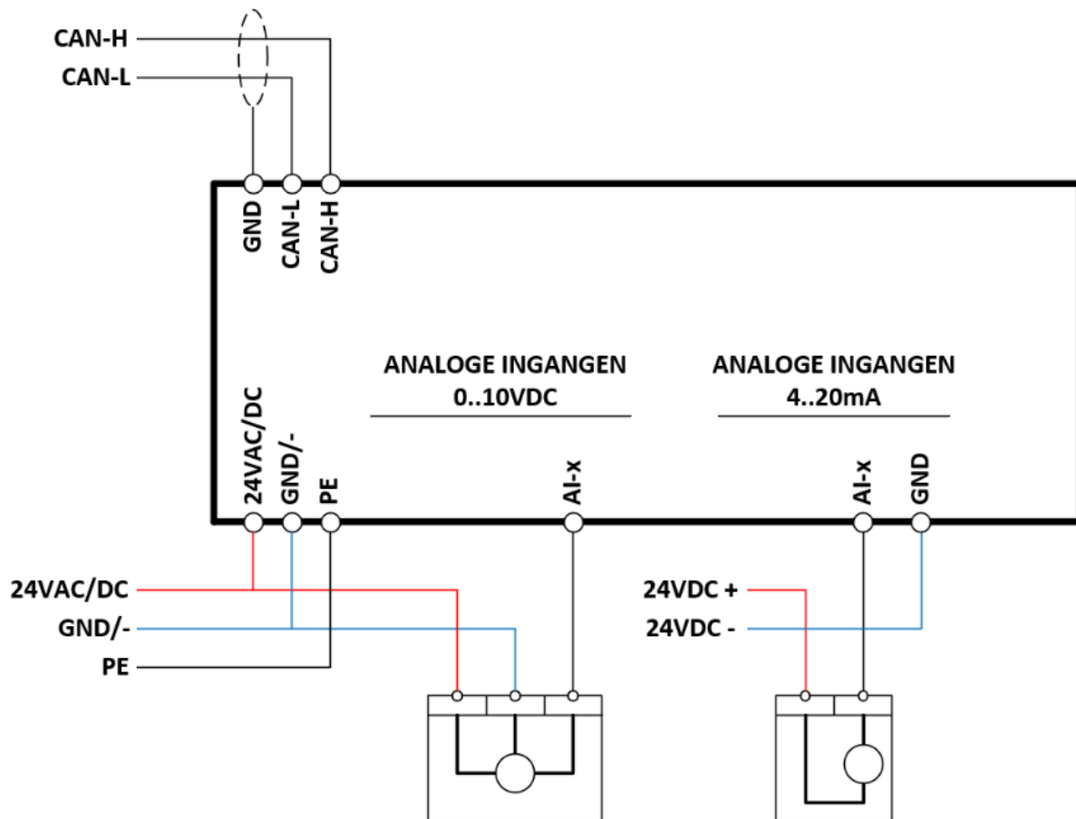
Figuur 2: Aansluitingen Analoge Ingangen
