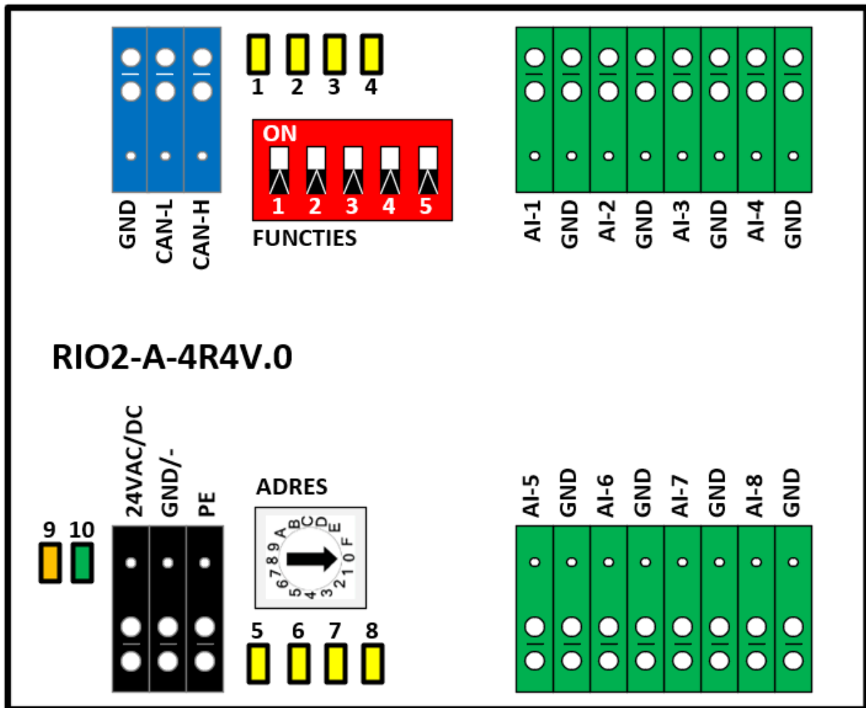
Figuur 1: Overzicht
