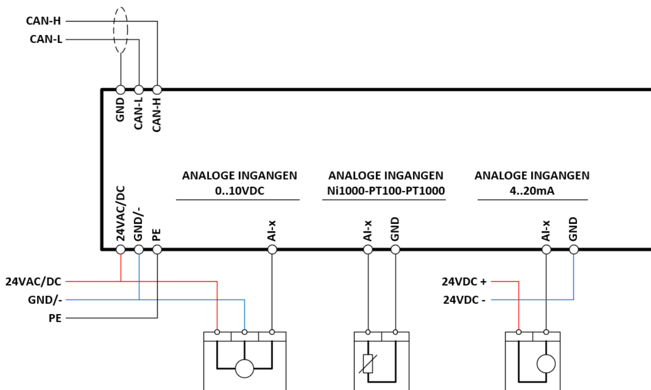
Figuur 2: Aansluitingen
