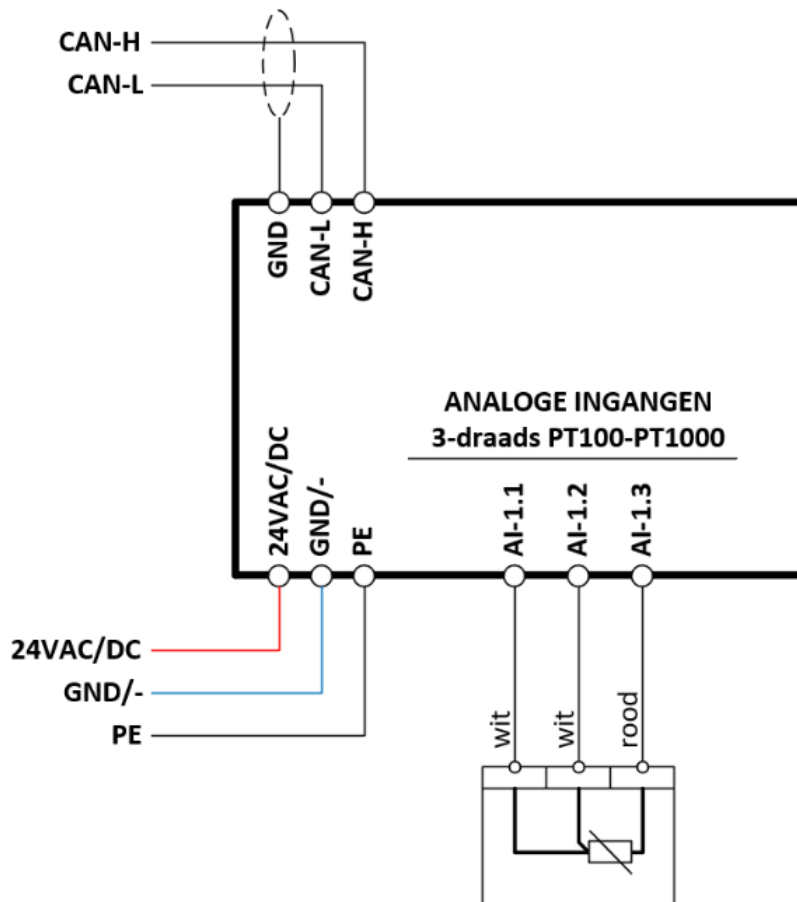
Figuur 2: Aansluitingen
