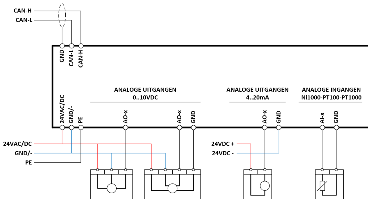
Figuur 3: Aansluitingen
