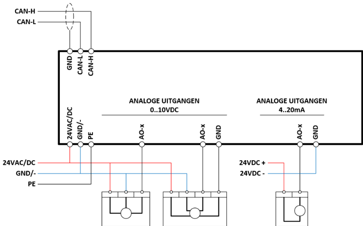
Figuur 2: Aansluitingen
