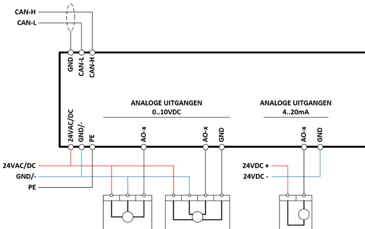
Figuur 2: Aansluitingen
