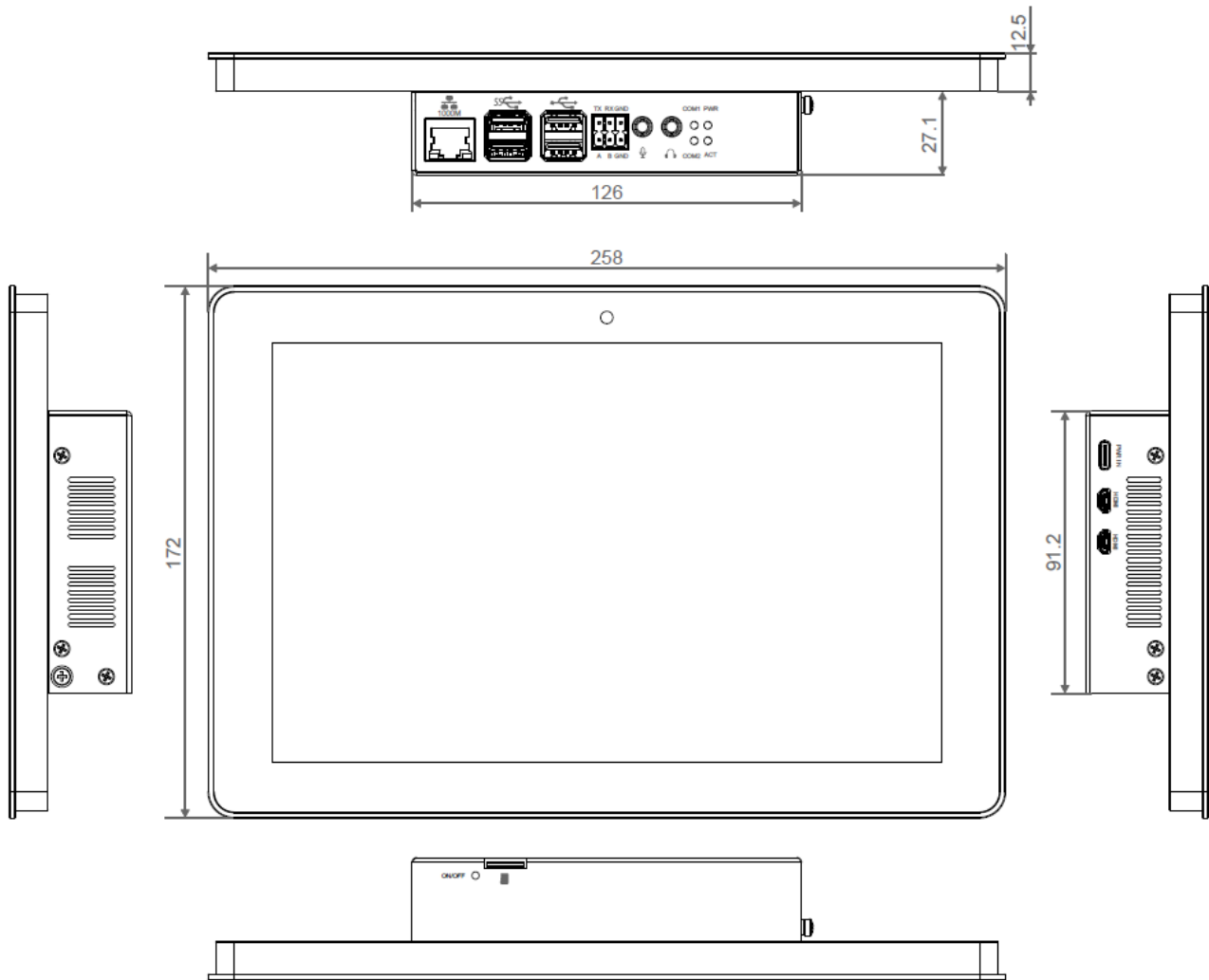
Figuur 1: Afmetingen
