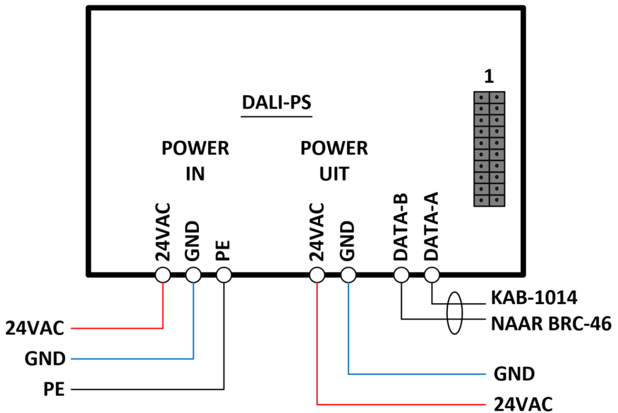
Figuur 3: Aansluitingen
