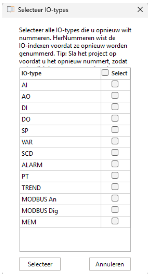
Figuur 35: Hernummeren
