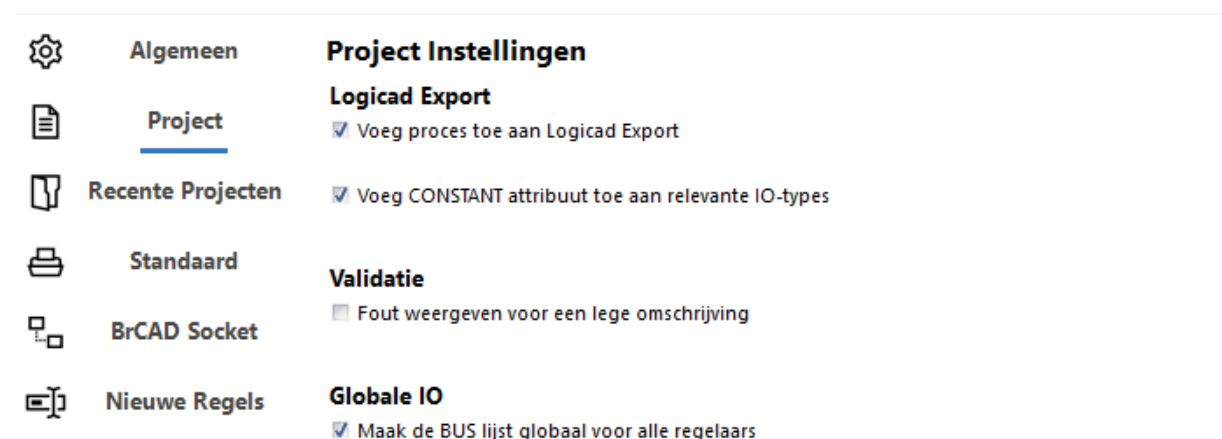
Figuur 81: Projectinstellingen
