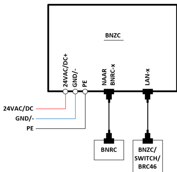
Figuur 2: Aansluitschema
