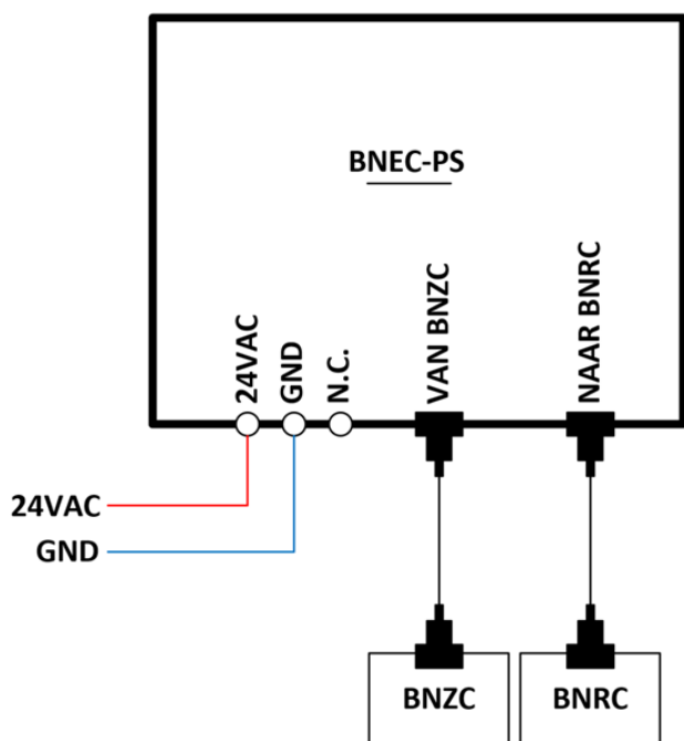
Figuur 2: Aansluitingen
