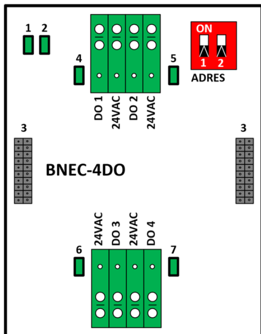
Figuur 2: Overzicht
