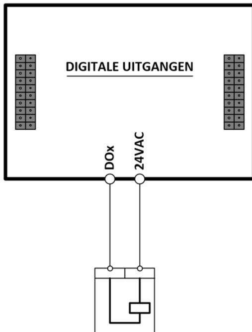
Figuur 3: Aansluitingen
