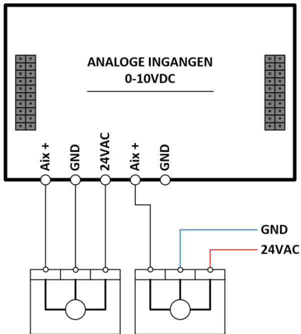
Figuur 3: Aansluitingen
