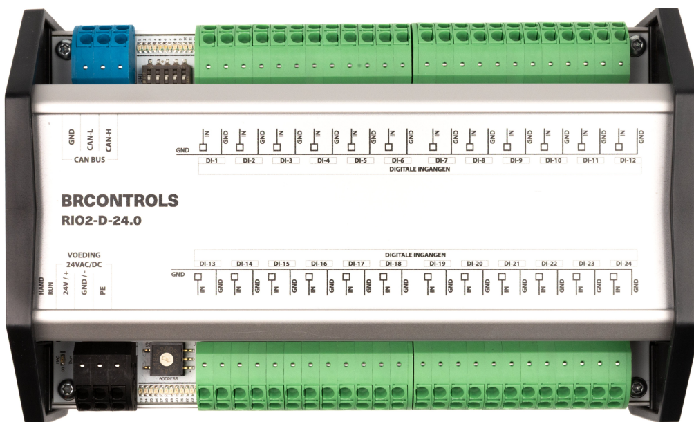
Afb 1: Bovenaanzicht
