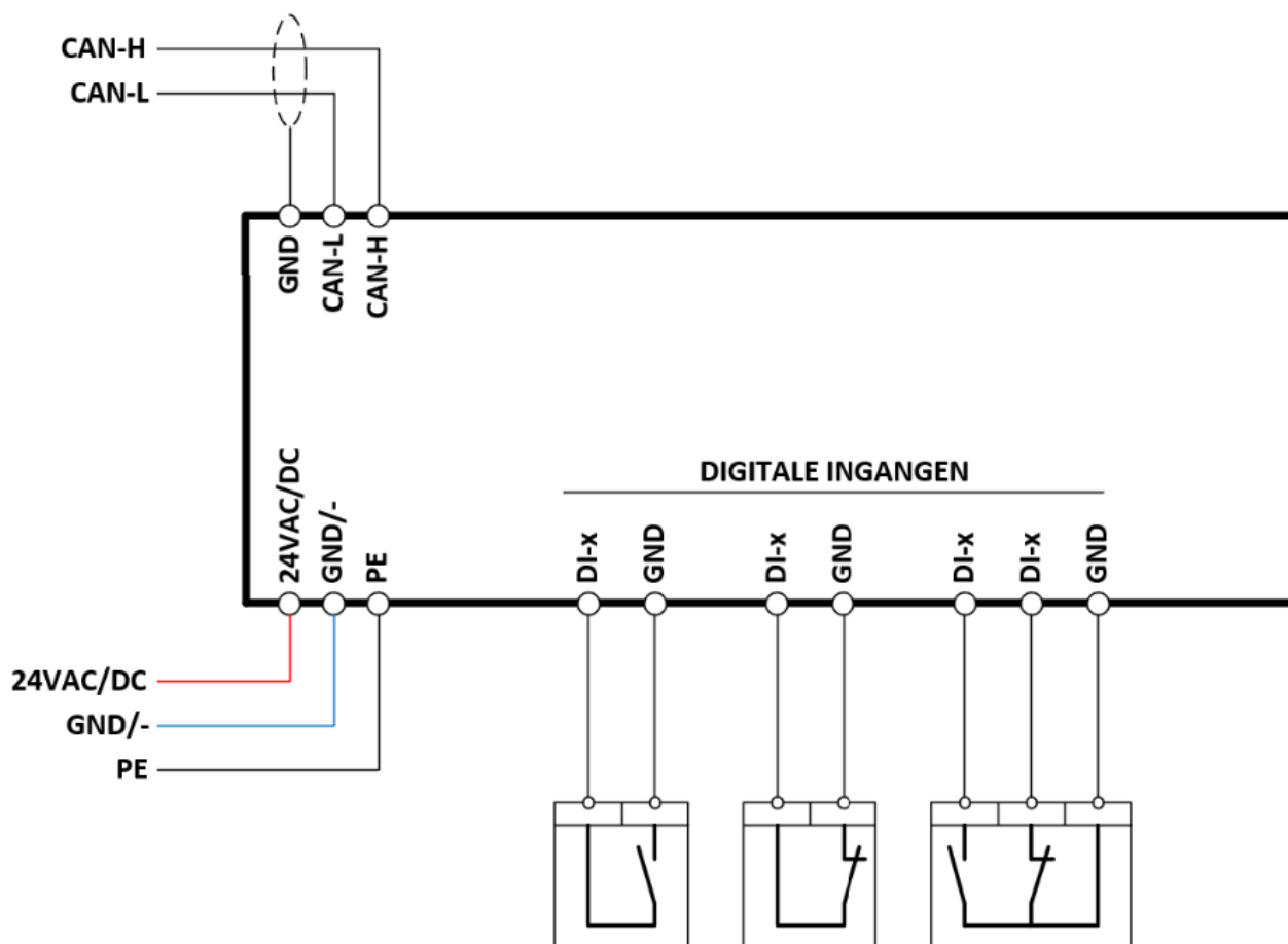
Afb 3: Aansluitschema
