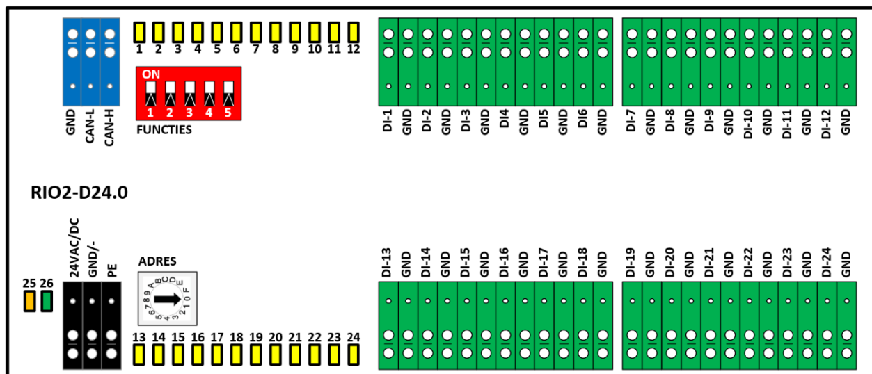
Afb 2: Overzicht LED's en aansluitingen
