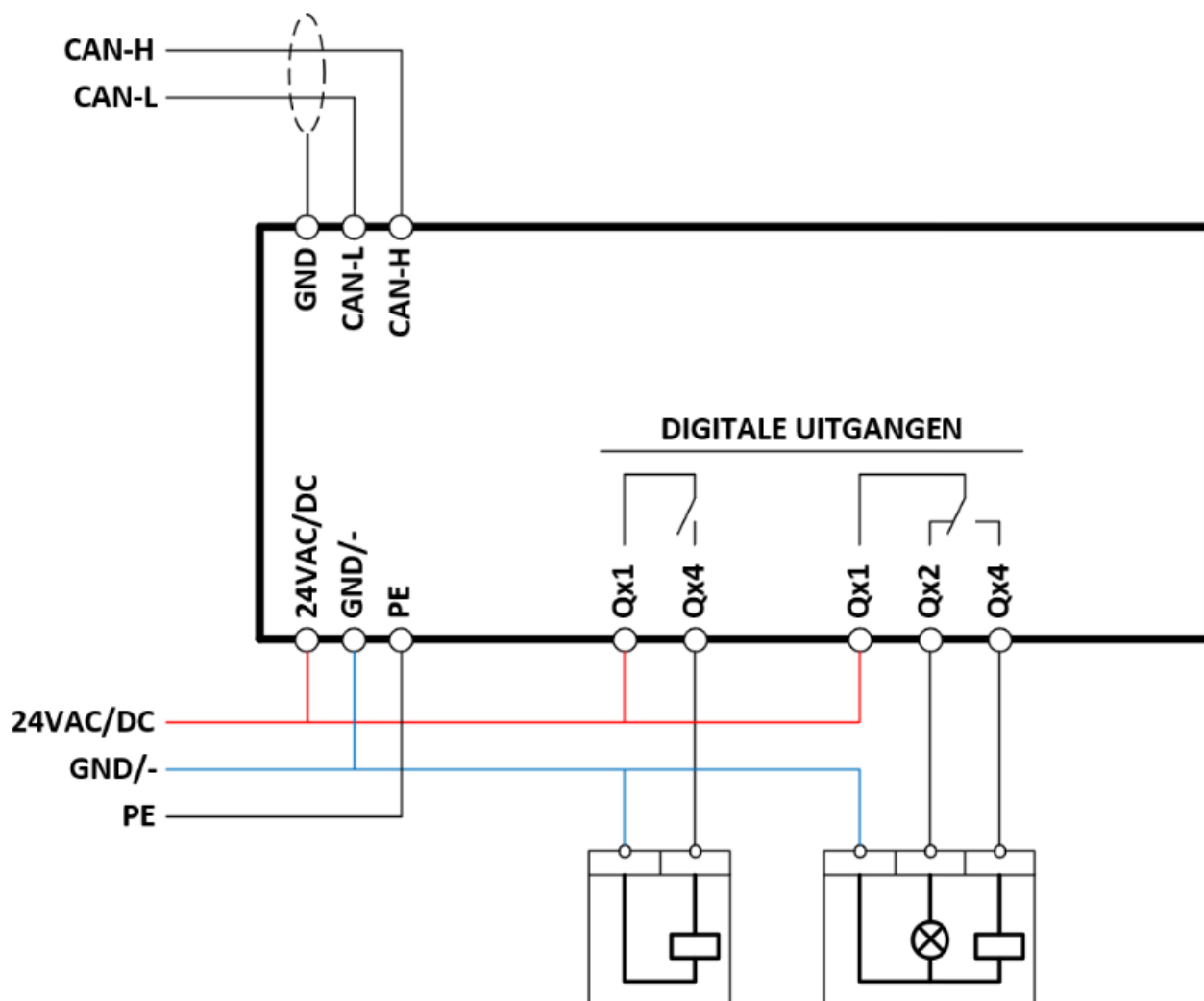
Afb 4: Aansluitschema
