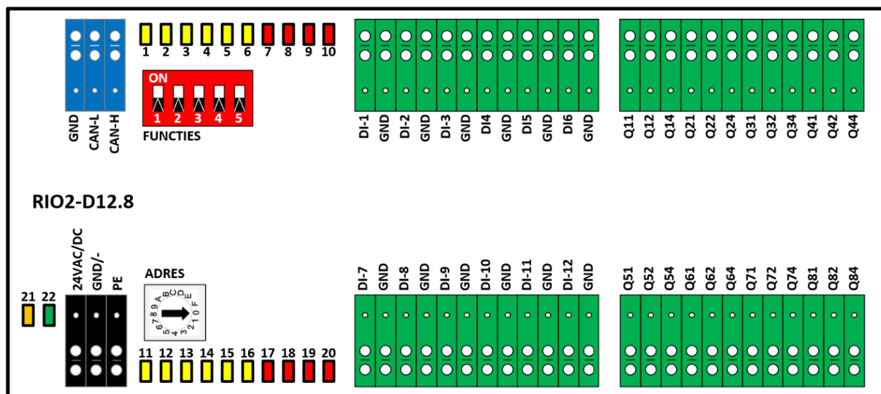
Afb 2: Overzicht LED's en aansluitingen
