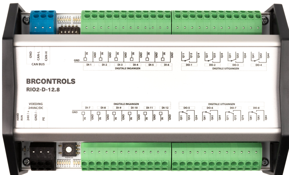
Afb 1: Bovenaanzicht
