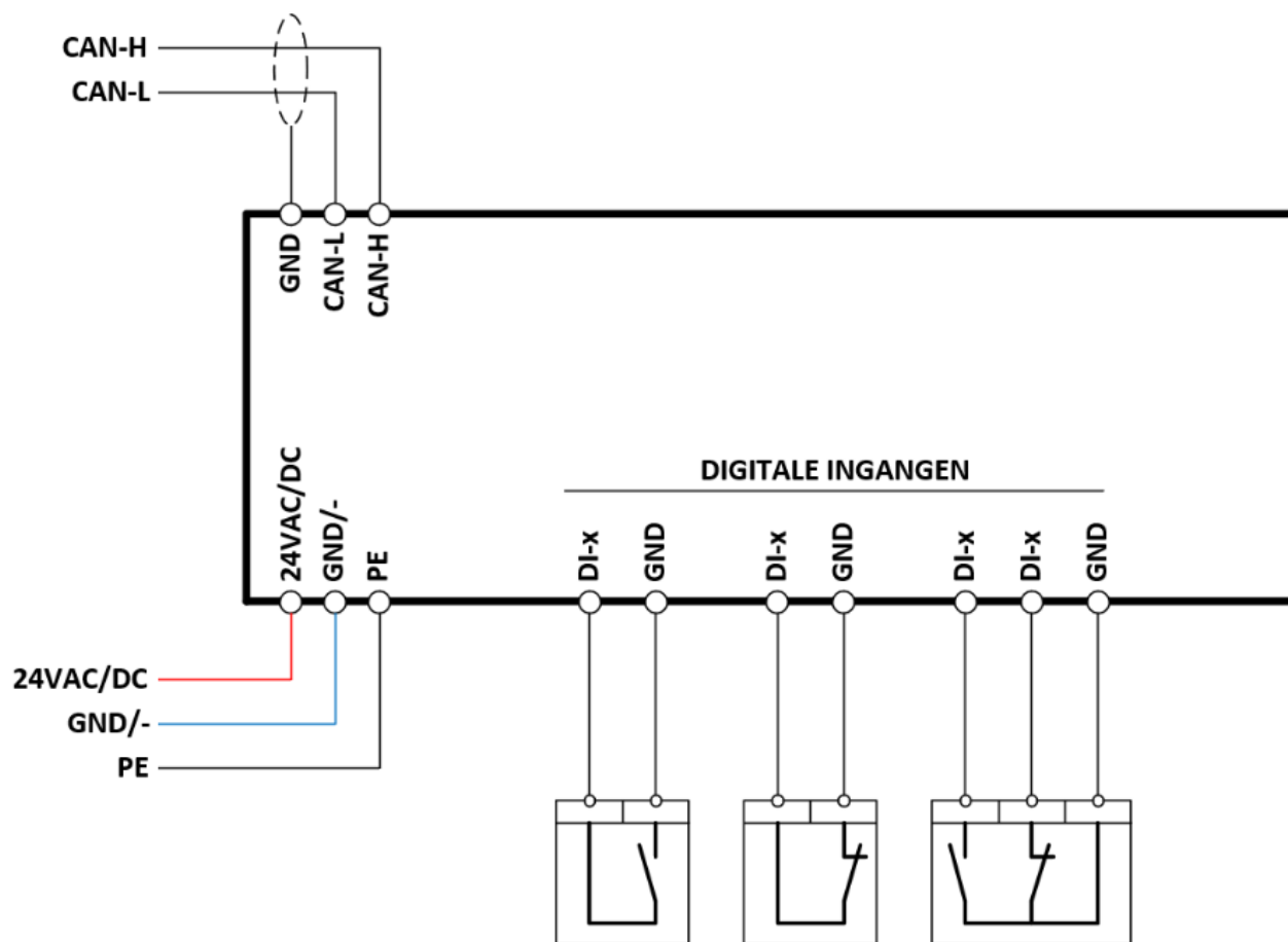
Afb 3: Aansluitschema
