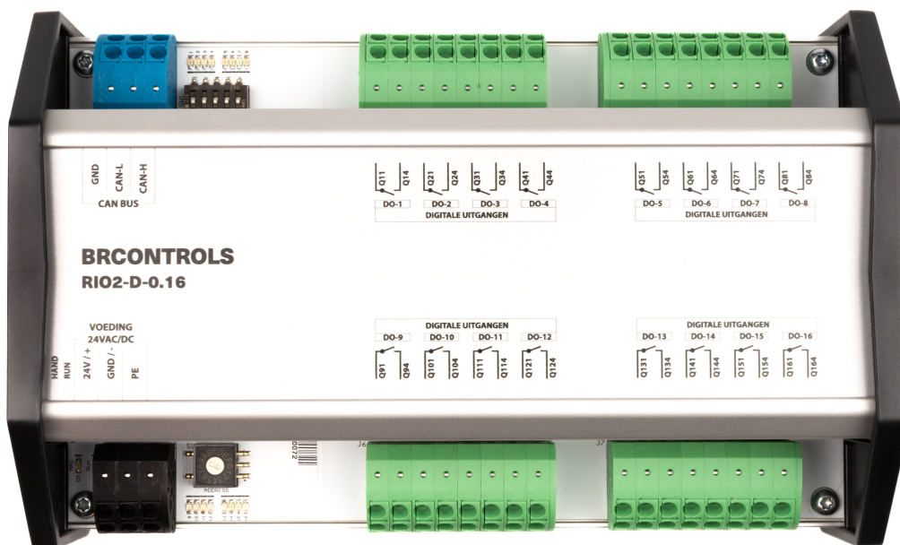
Afb 1: Bovenaanzicht
