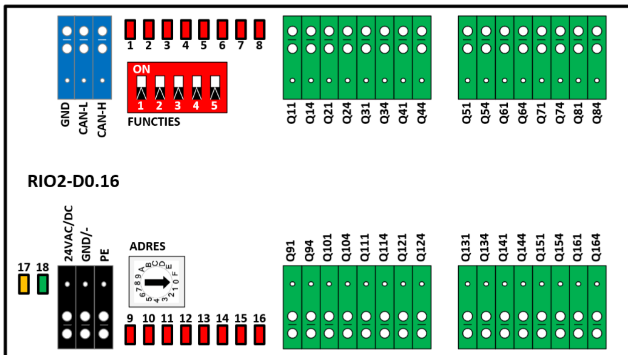
Afb 2: Overzicht LED's en aansluitingen
