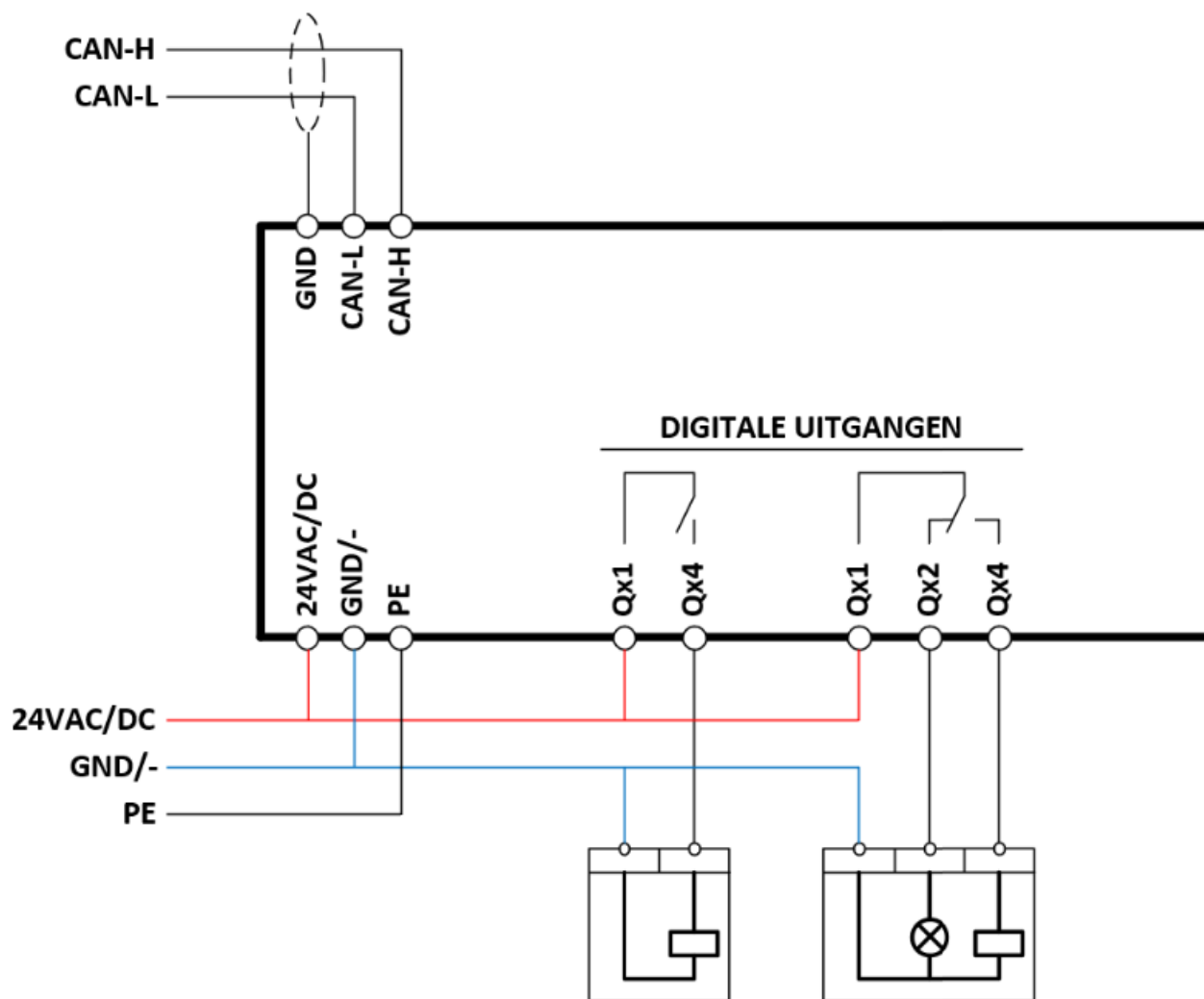
Afb 3: Aansluitschema
