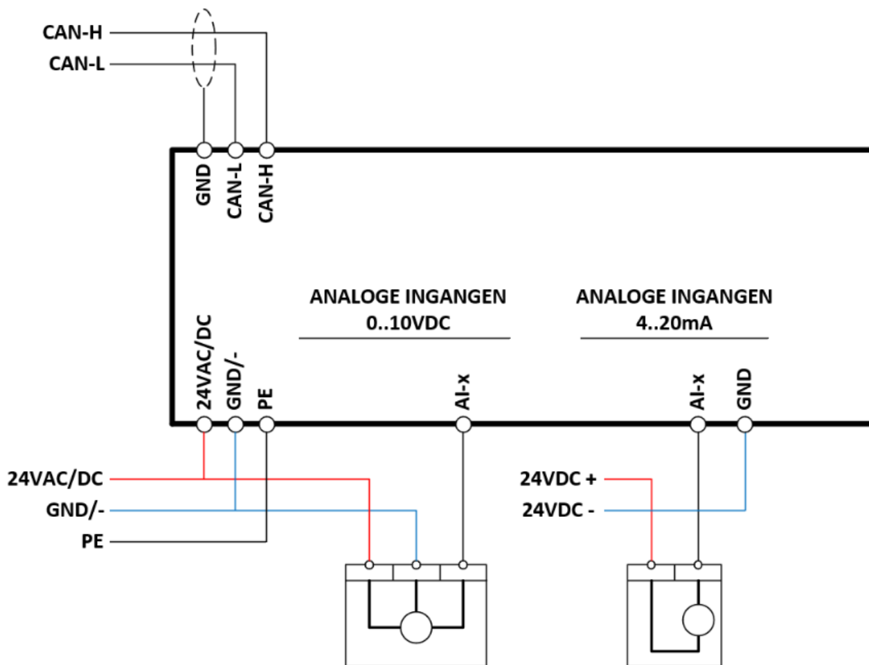
Afb 3: Aansluitschema
