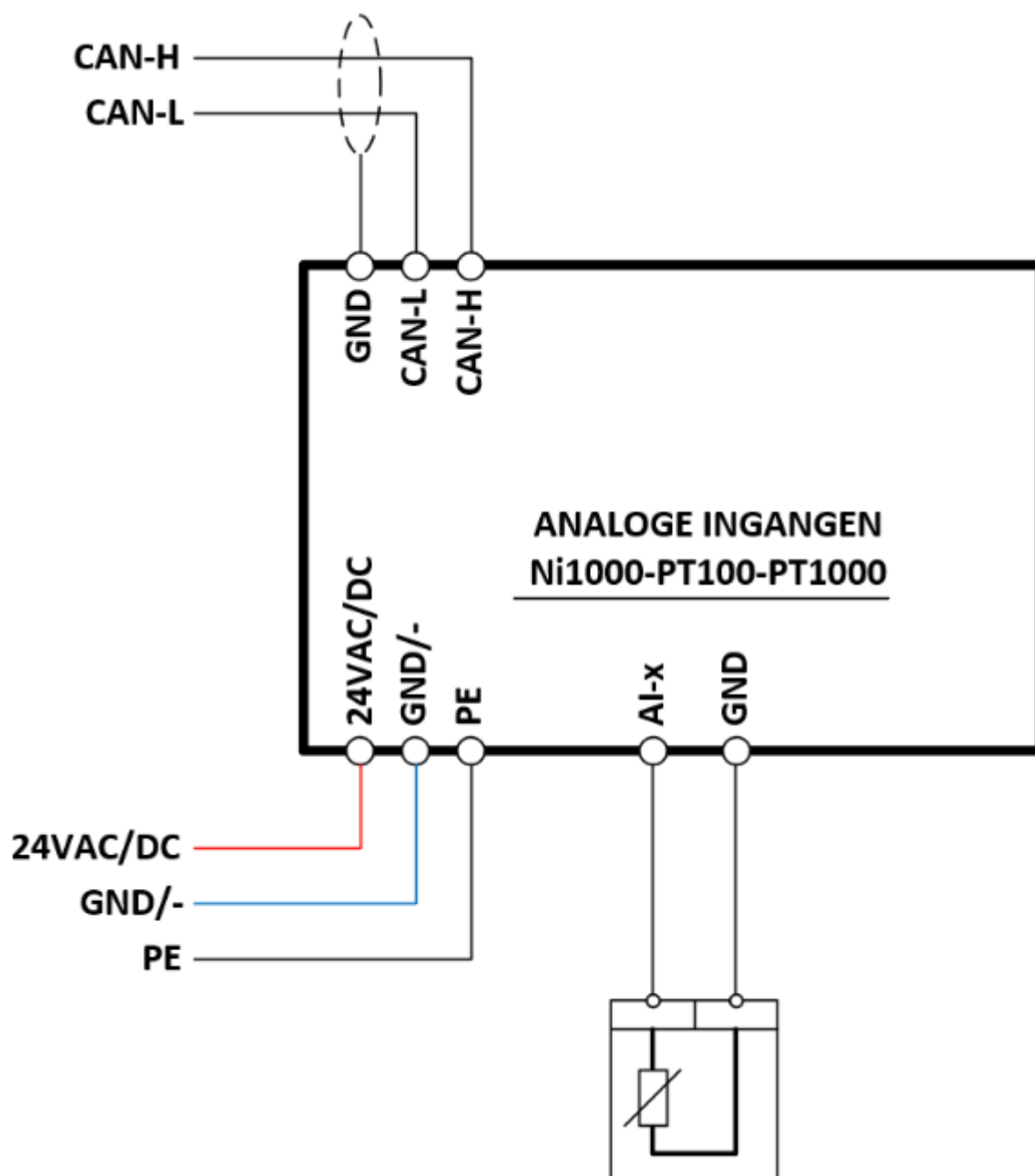
Afb 3: Aansluitschema
