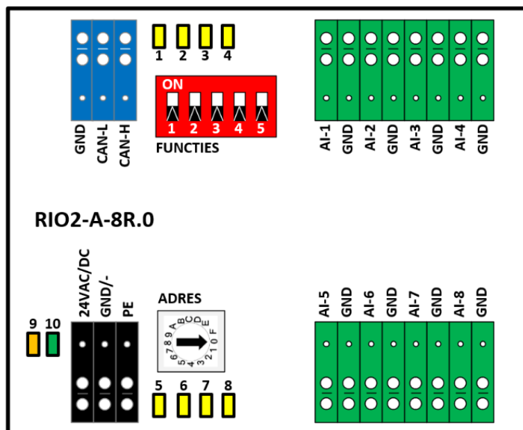
Afb 2: Overzicht LED's en aansluitingen
