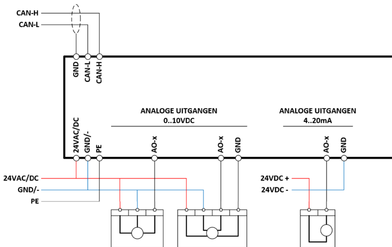
Afb 3: Aansluitschema
