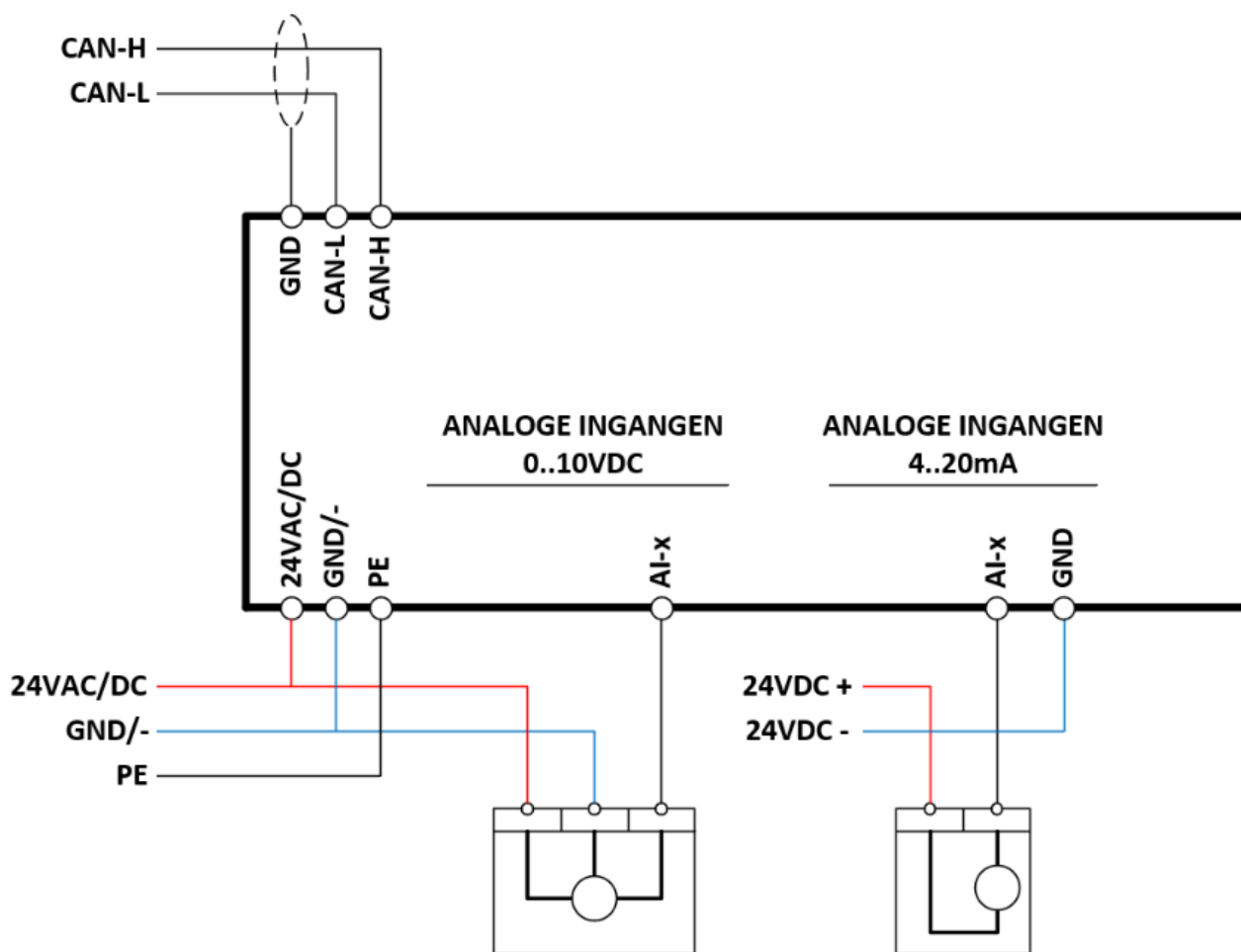
Afb 2: Aansluitschema
