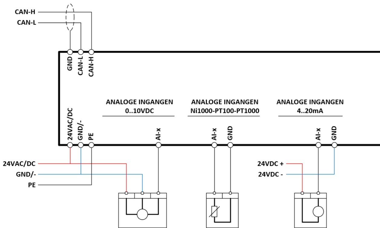
Afb 3: Aansluitschema
