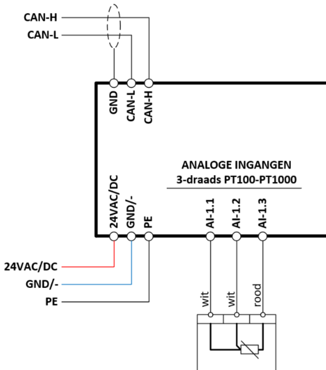
Afb 2: Aansluitschema
